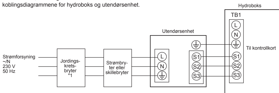
<Figur 4.4.2> Elektriske koblinger 1-fase
