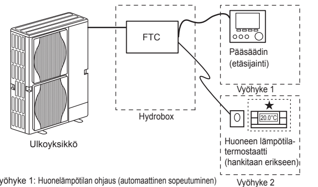
Vyöhyke 1: Huonelämpötilan ohjaus (automaattinen sopeutuminen) Vyöhyke 2: Lämpökäyrä tai virtauslämpötilan ohjaus
