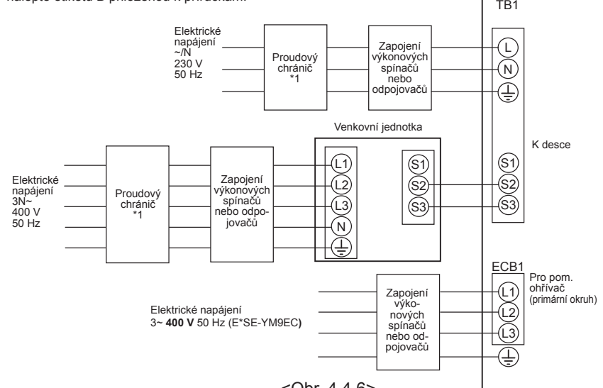
<Obr. 4.4.6> Elektrické přívody, 3fázové
