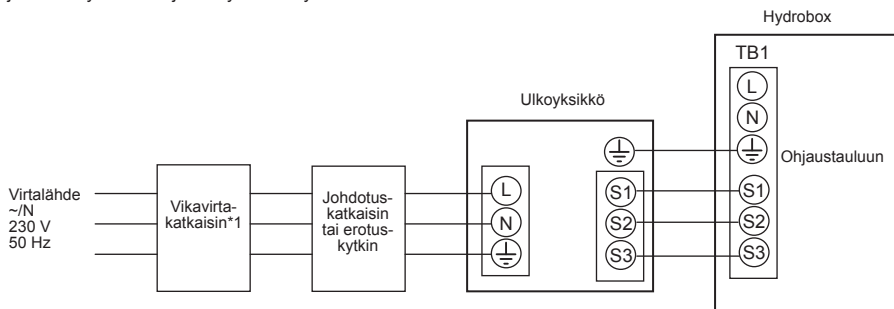
<Kuva 4.4.2> Sähkölaitännät, 1-vaihe
