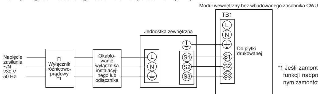
<Rysunek 4.4.2> Przyłącza elektryczne 1-fazowe
