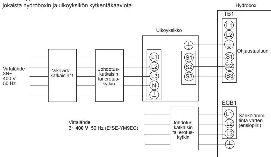
<Kuva 4.4.3> Sähkölaitännät, 3-vaihe
