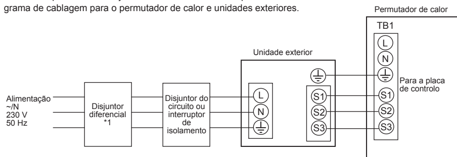
<Figura 4.4.2> Ligações eléctricas para alimentação monofásica
