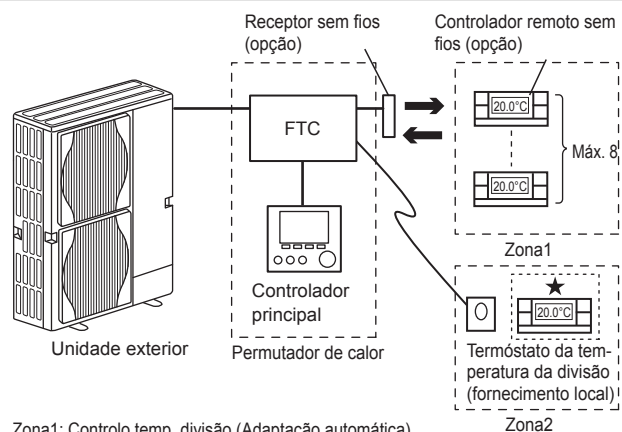
Zona1: Controlo temp. divisão (Adaptação automática) Zona2: Curva de compensação ou controlo temp. caudal
