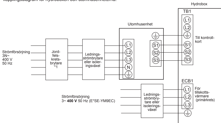
<Bild 4.4.3> Elanslutningar 3-fas
