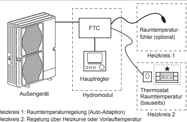
Heizkreis 1: Raumtemperaturregelung (Auto-Adaption) Heizkreis 2: Regelung über Heizkurve oder Vorlauftemperatur
