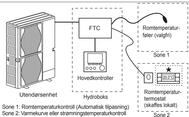
Sone 1: Romtemperaturkontroll (Automatisk tilpasning) Sone 2: Varmekurve eller strømningsstemperaturkontroll
