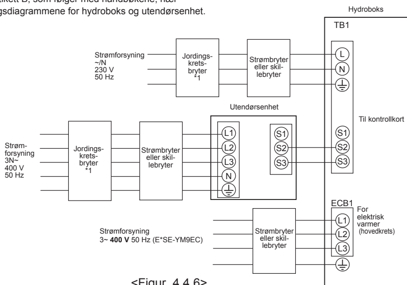
<Figur 4.4.6> Elektriske koblinger 3-fase
