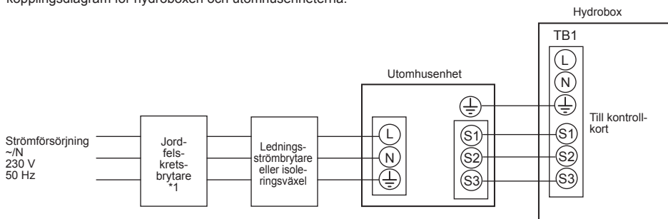
<Bild 4.4.2> Elanslutningar 1-fas
