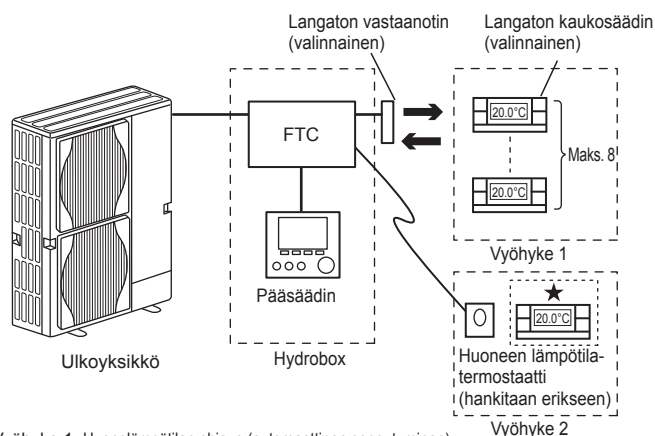
Vyöhyke 1: Huonelämpötilan ohjaus (automaattinen sopeutuminen) Vyöhyke 2: Lämpökäyrä tai virtauslämpötilan ohjaus
