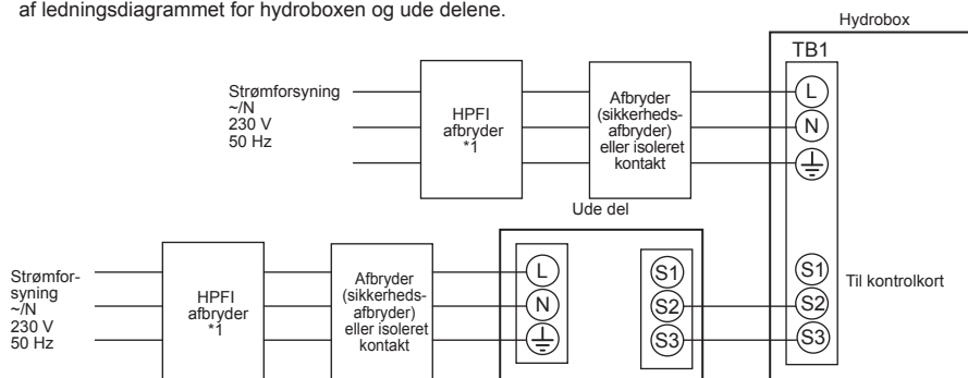
<Figur 4.4.5> Elektriske tilslutninger 1 - faset
