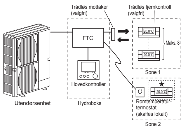
Sone 1: Romtemperaturkontroll (Automatisk tilpasning) Sone 2: Varmekurve eller strømningsstemperaturkontroll
