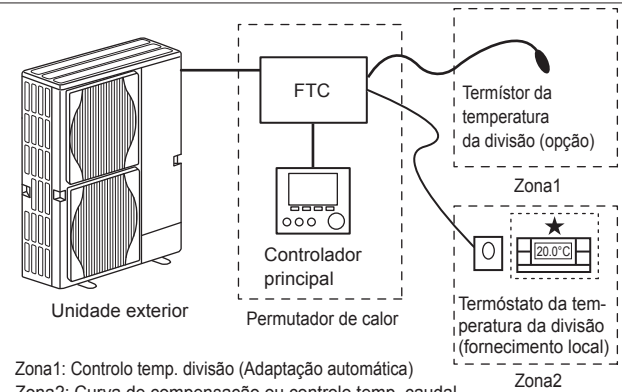
Zona1: Controlo temp. divisão (Adaptação automática) Zona2: Curva de compensação ou controlo temp. caudal
