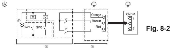
Fig. 8-2 A Beispiel eines Schaltplans (Anforderungsfunktion) B Anordnung vor Ort C Externer Eingangsadapter (PAC-SC36NA-E) D Schalttafel der Außenanlage E Max. 10 m F Stromversorgung für Relais X, Y: Relais
