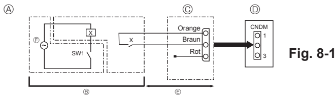
Fig. 8-1 A Beispiel eines Schaltplans (Lärmschutzmodus) B Anordnung vor Ort C Externer Eingangsadapter (PAC-SC36NA-E) D Schalttafel der Außenanlage E Max. 10 m F Stromversorgung für Relais X: Relais
