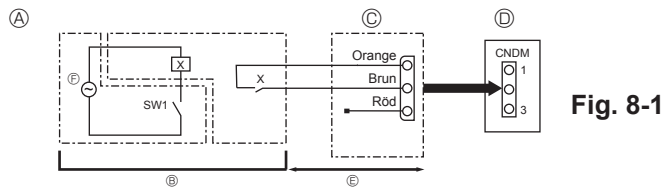
Fig. 8-1 Ⓐ Exempel på kopplingsschema (lägsta ljud-nivå) Ⓓ Utomhusenhetens kontrollkort Ⓑ Uppställning på plats Ⓔ Max. 10 m Ⓒ Yttre inadaptor (PAC-SC36NA-E) Ⓕ Strömförsörjning för rela X: Relä
