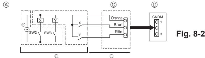
Fig. 8-2 Ⓐ Exempel på kopplingsschema (Behovsfunktion) Ⓒ Yttre inadaptor (PAC-SC36NA-E) Ⓑ Uppställning på plats Ⓓ Utomhusenhetens kontrollkort X, Y: Relä Ⓔ Max. 10 m Ⓕ Strömförsörjning för rela
