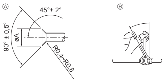
Ⓐ Διαστάσεις εκχειλίωσης Ⓑ Ροπή σύσφιξης για το περικόχλιο εκχειλίωσης
