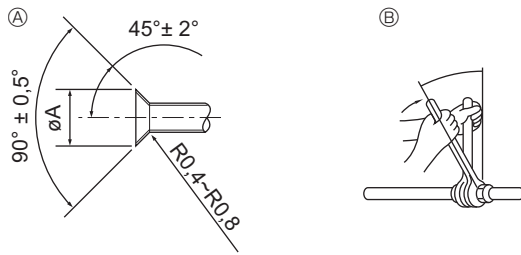
Ⓐ Afsnijmaten tromp Ⓑ Aanhaalmoment flensmoer
