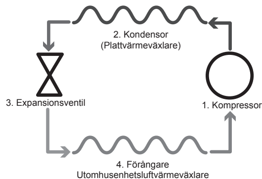
Schema över enhetscylindersystem
