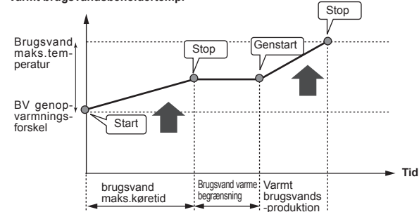
Varmt brugsvandsbeholdertemp.
